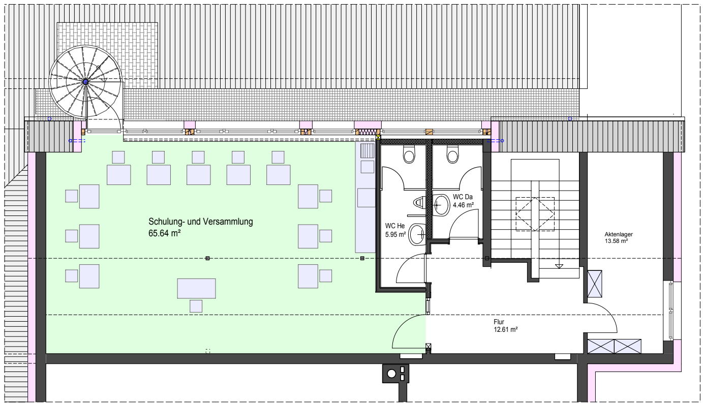
GRUNDRISS 1. OG
